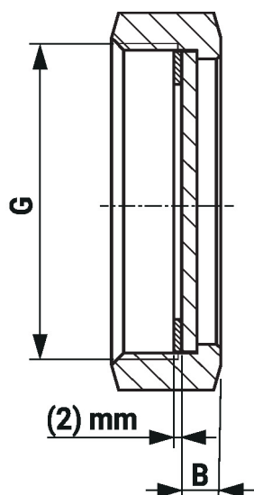
Rysunki wymiarowe
