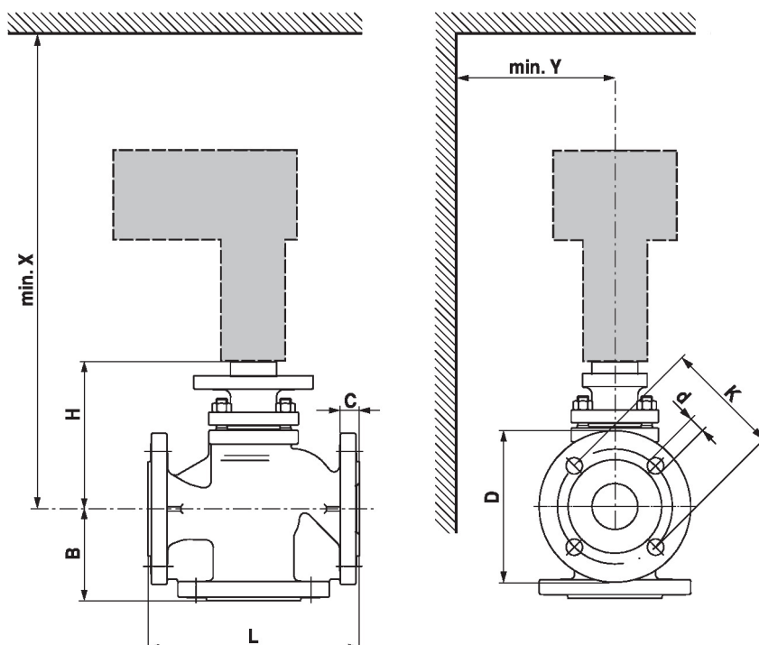
Rysunki wymiarowe
