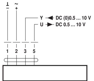
NRF24A-SZ(-0) SRF24A-SZ(-0)
