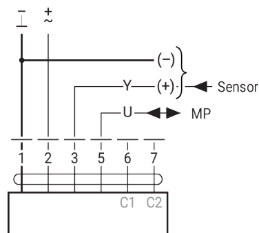
MP-Bus
