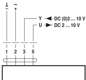
NRF24A-SR(-0) SRF24A-SR(-0)
