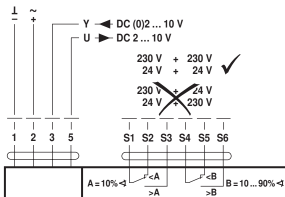
NRF24A-SR-S2(-0) SRF24A-SR-S2(-0)
