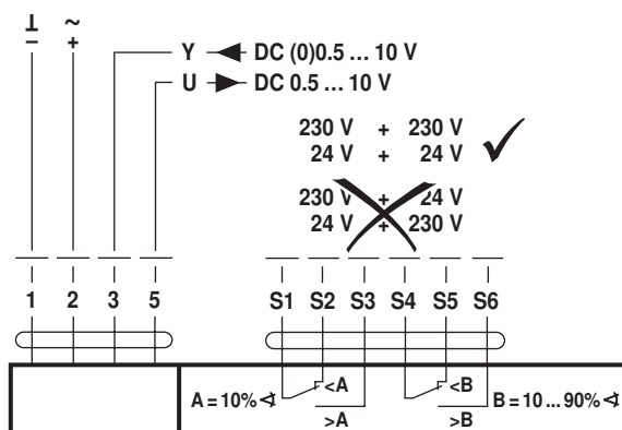
NRF24A-SZ-S2(-0) SRF24A-SZ-S2(-0)
