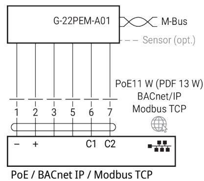
BACnet IP / Modbus TCP
