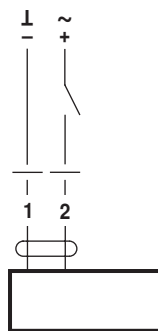
NRF24A(-O) SRF24A(-O)
