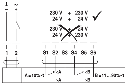
NRF24A-S2(-O) SRF24A-S2(-O)
