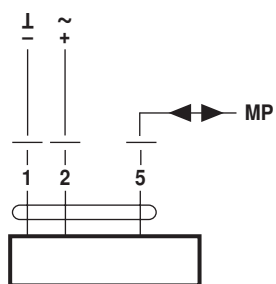
CM24-MPL-F..
