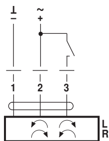
CM24-F..
