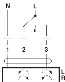
CM230-F..
