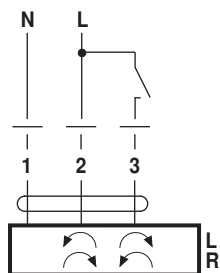
CM230-F..
