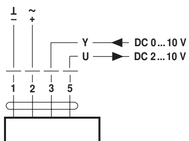
CM24-SR-F..
