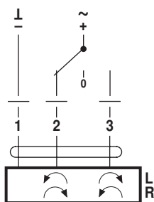
CM24-F..
