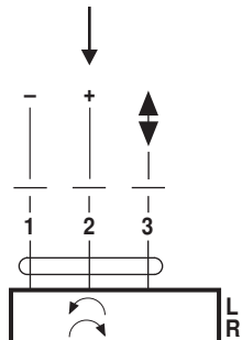
CM24K-F-T..
