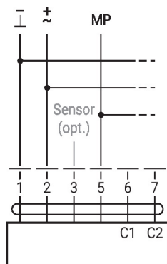
Szyna MP-Bus, zasilanie poprzez przyłącze 3-przewodowe
