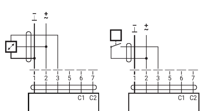
Połączenie z czujnikiem aktywnym Połączenie z zestykiem
