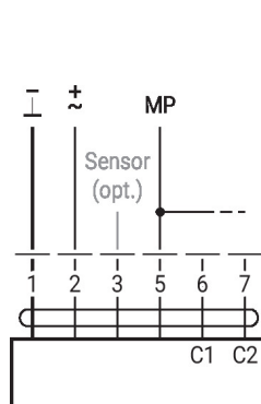
Szyna MP-Bus poprzez przyłącze 2-przewodowe, zasilanie lokalne
