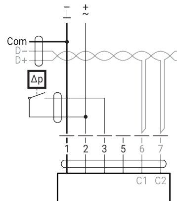
MP-Bus
