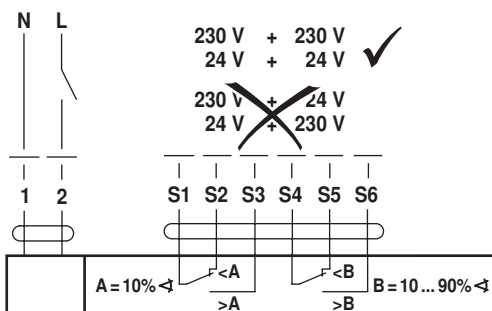
EF230A-S2 / EF230G-S2
