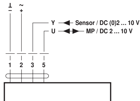
EF24A-MP / EF24G-MP
