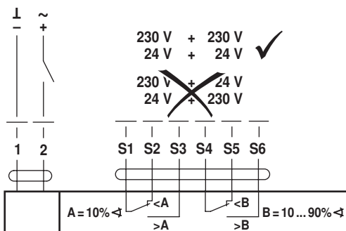
EF24A-S2 / EF24G-S2
