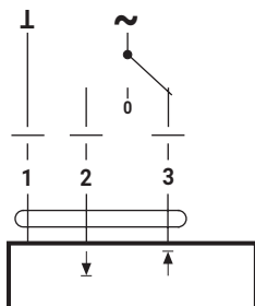
NRDVX24-3-T..
