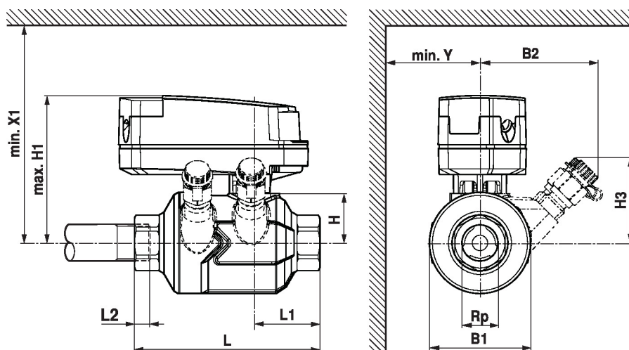
Rysunki wymiarowe
