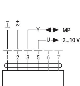
MP-Bus
