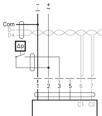
MP-Bus
