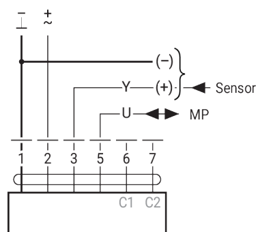
MP-Bus
