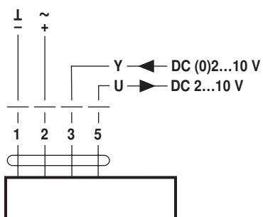
GR24A-SR-R / GR24A-MF-R
