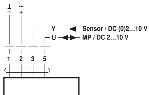
GR24A-MP-R
