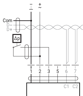
MP-Bus
